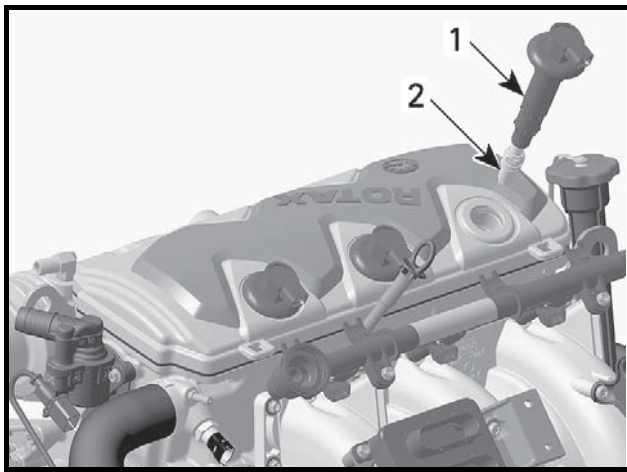
1. Катушка зажигания
