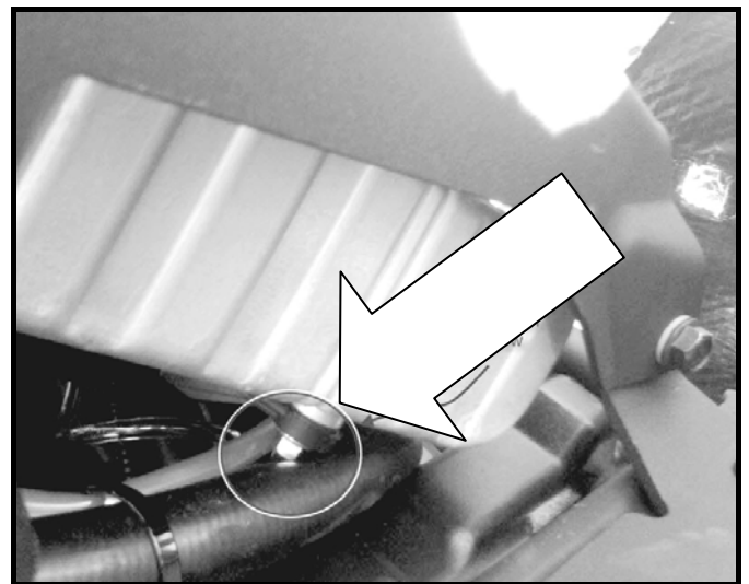
Сместите шланг внутрь. Шланг не должен касаться болта.
