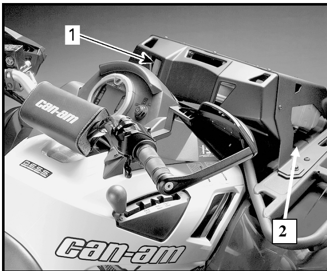
1 – радиатор 2 – место контроля положения шланга
