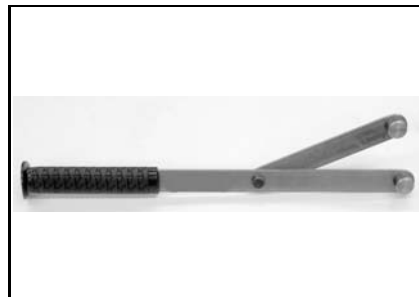
Pulley Holder P/N 529 036 054 Recommended Rally, DS 250, DS 70/90
