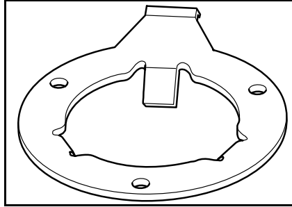
Fan holder tool P/N 529 036 006 Mandatory 552F
